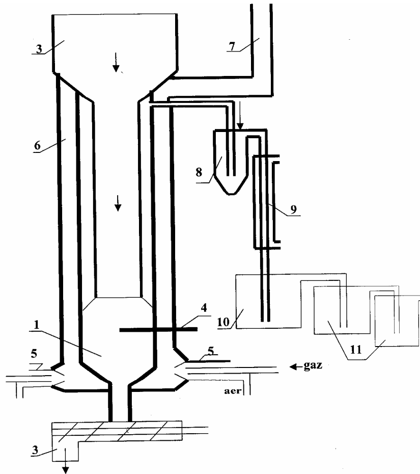
Schema instalației pentru denocivirea deșeurilor viticole ce conțin albastru de Prusia
